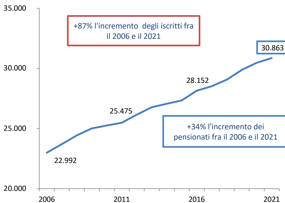
Fig. 6 – Numero delle pensioni vigenti, 2006-2021 (v.a.)
