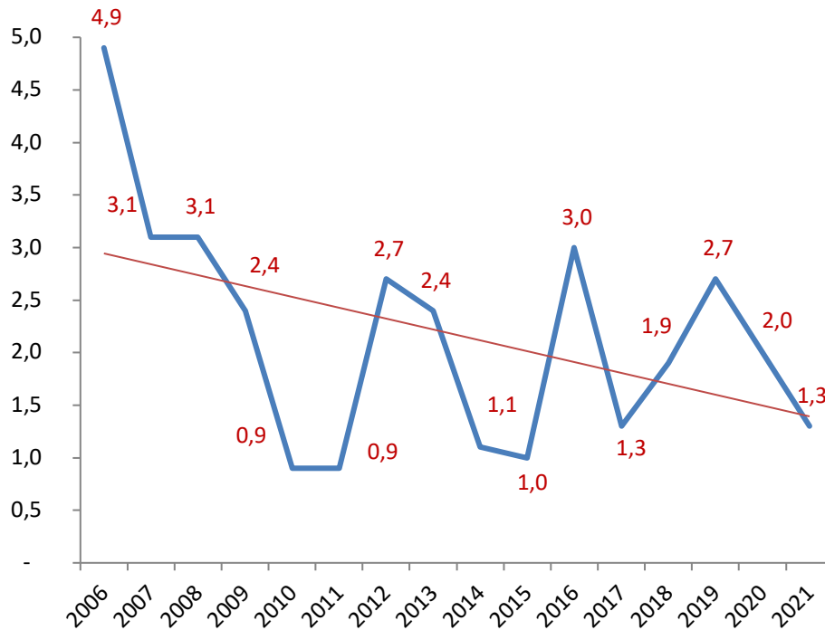
Fig. 7 – Tasso annuo di crescita delle pensioni vigenti, 2006 - 2021 (var.% sull'anno precedente)
